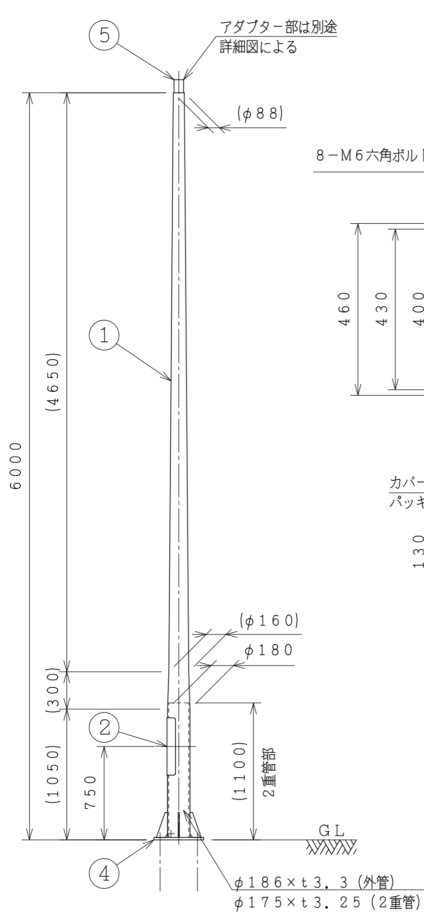
ポール姿図 S=1:30
