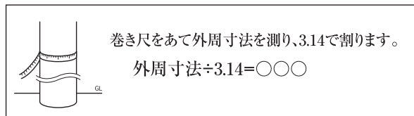
図5. 外周寸法
