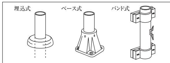
図2. 根元詳細
