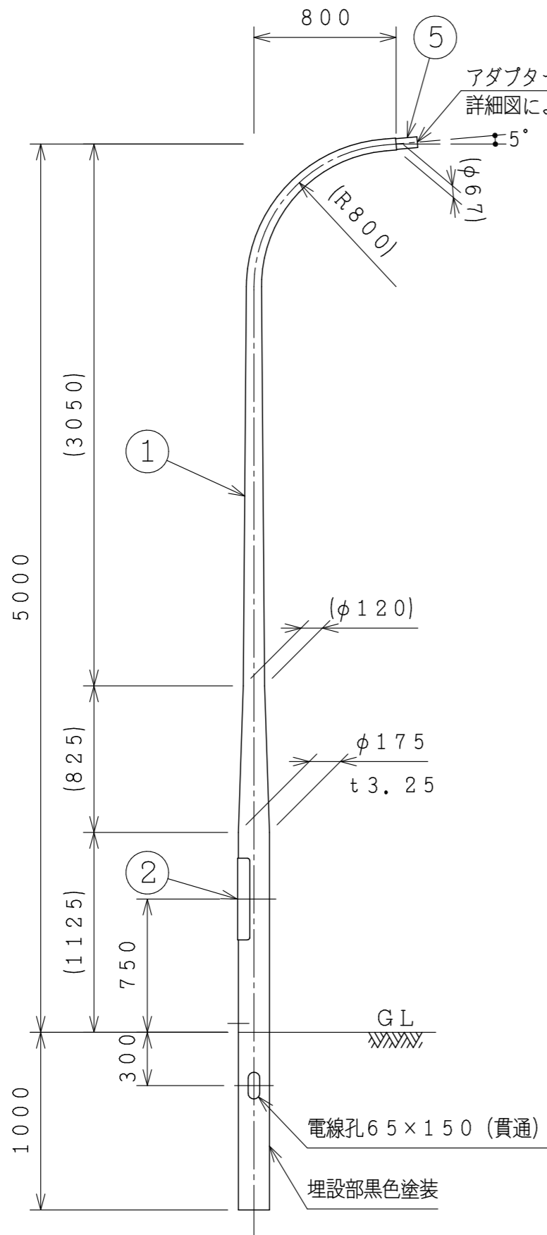
ポール姿図 S=1:30
