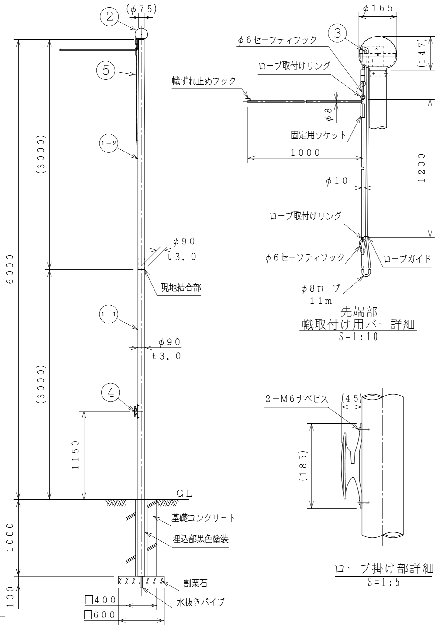
ポール姿図 S=1:30
